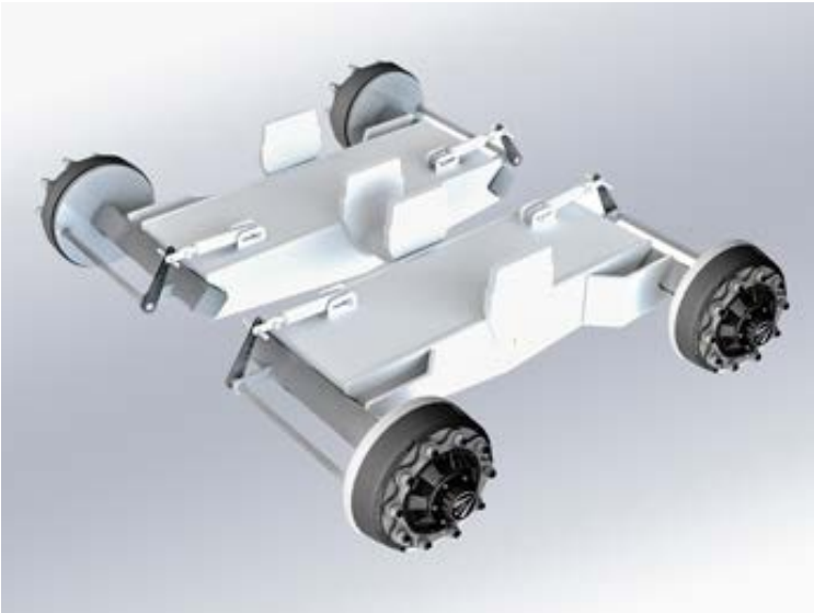
Eje balancín cuadrado 100mm, vía 1900, 10 esp., tambor freno 400x80.
