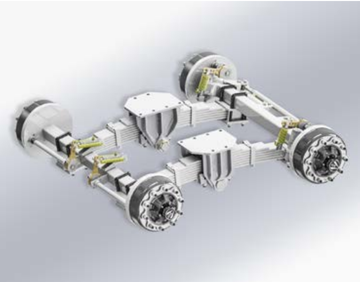
Disponible de 100mm en modelos E88KMP2 y E92KMP2. Disponible de 150mm en modelos E94KMP2 y E95KMP2. De serie: Eje suspensión bogie autodireccional en segundo eje cuadrado 100 o 150mm, vía 2000, 10 esp., tambor freno 400x120. En opción: Eje suspensión bogie direccional forzado en segundo eje cuadrado 100 o 150mm comandado con cilindro enganchado al tractor, vía 2000, 10 esp., tambor freno 400x120. Según norma ISO 26402. Eje suspensión bogie direccional forzado en segundo eje cuadrado 100 o 150mm comandado electrónicamente, vía 2000, 10 esp., tambor freno 400x120.
