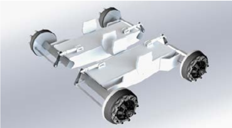
Disponible de 100mm en modelos E88KMP2 y E92KMP2. Disponible de 150mm en modelos E94KMP2 y E95KMP2. De serie: Eje suspensión bogie autodireccional en segundo eje cuadrado 100 o 150mm, vía 2000, 10 esp., tambor freno 400x120. En opción: Eje suspensión bogie direccional forzado en segundo eje cuadrado 100 o 150mm comandado con cilindro enganchado al tractor, vía 2000, 10 esp., tambor freno 400x120. Según norma ISO 26402. Eje suspensión bogie direccional forzado en segundo eje cuadrado 100 o 150mm comandado electrónicamente, vía 2000, 10 esp., tambor freno 400x120.
